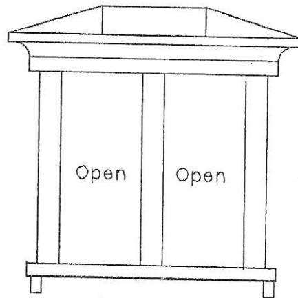
End Elevation
